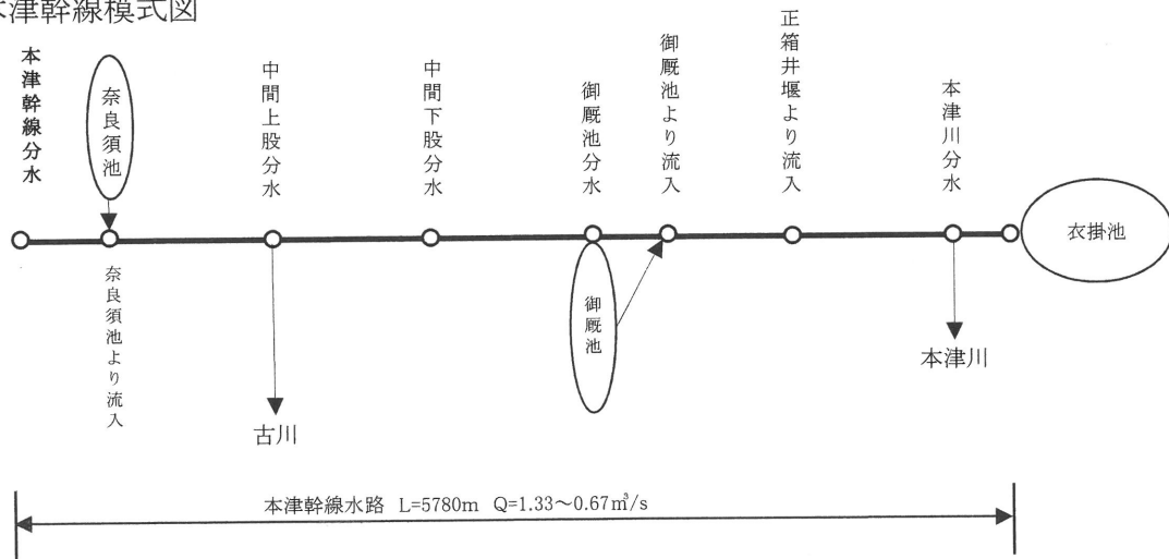
本津幹線模式図
