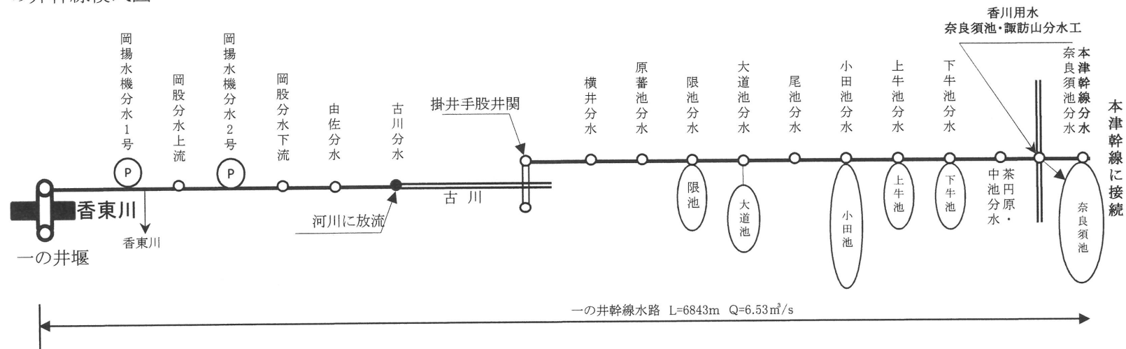
本津幹線模式図
