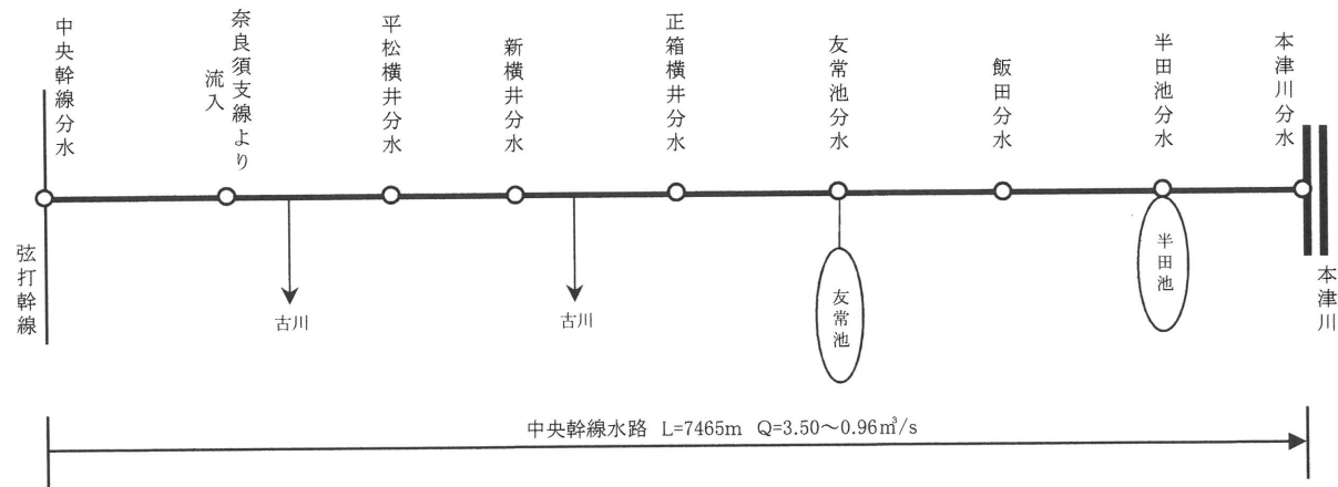
中央幹線模式図
