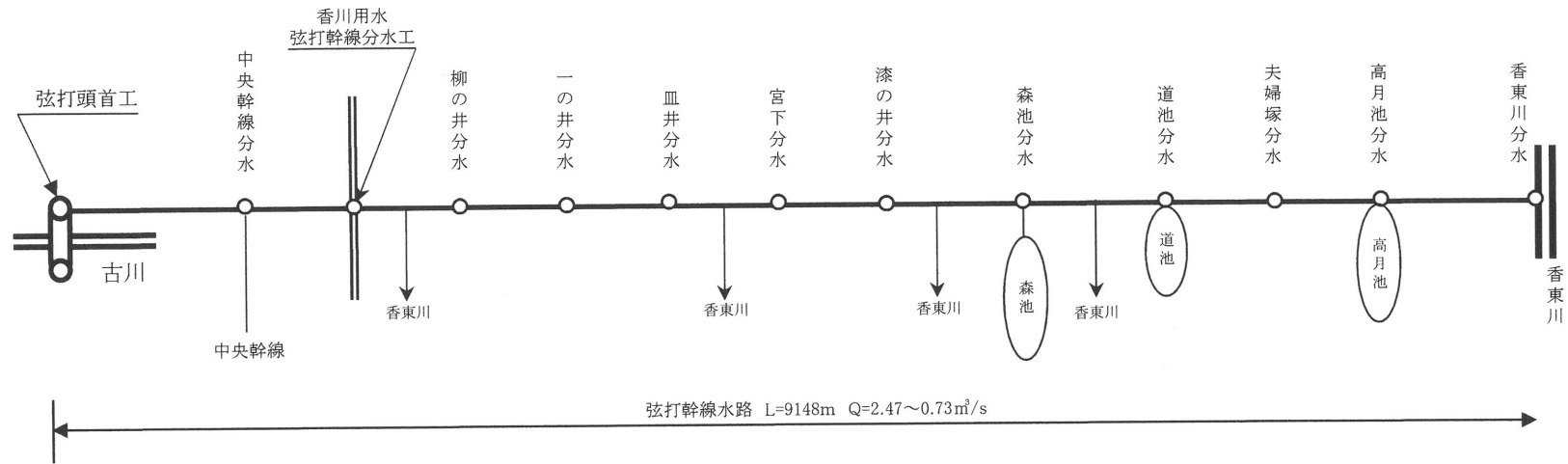
弦打幹線模式図
